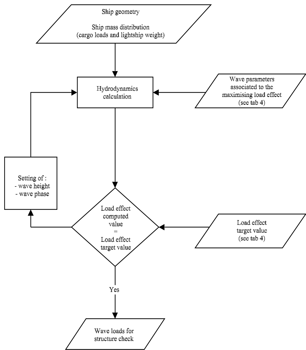
Figure 2 : Wave parameter calculations
